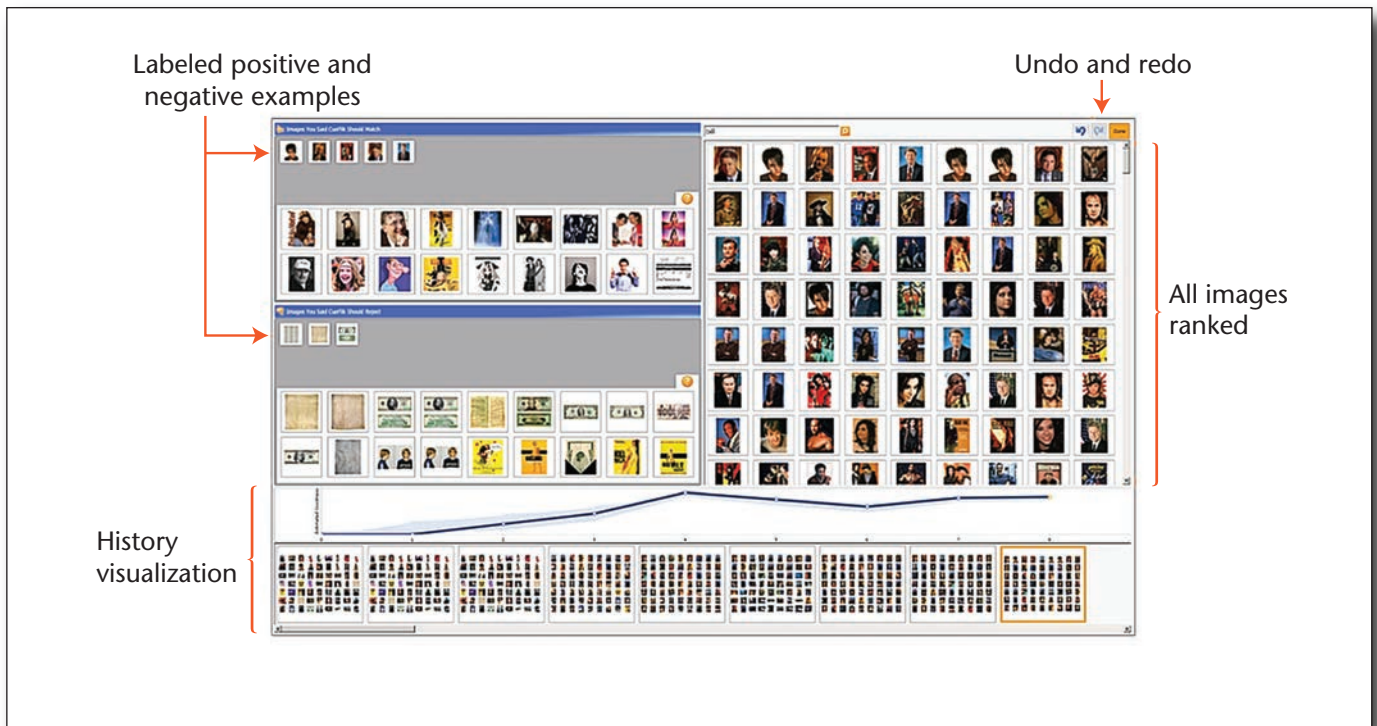
Figure 6. CueFlik.
