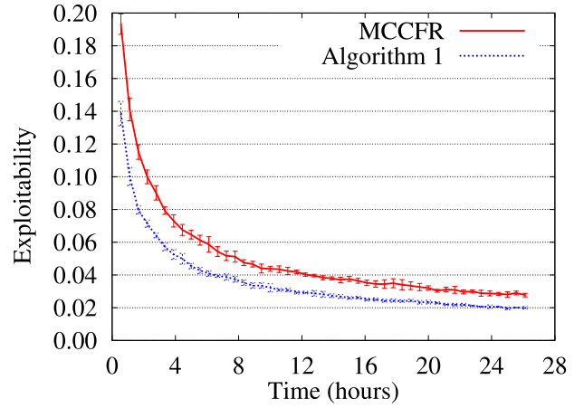
(a) Goofspiel(7)
