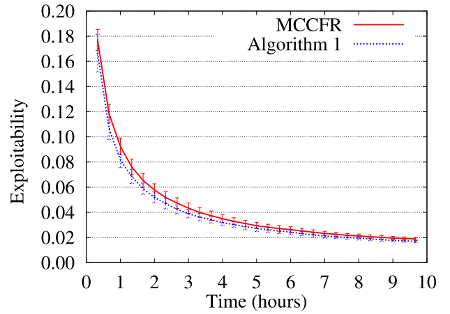
(b) Bluff(2,2)
